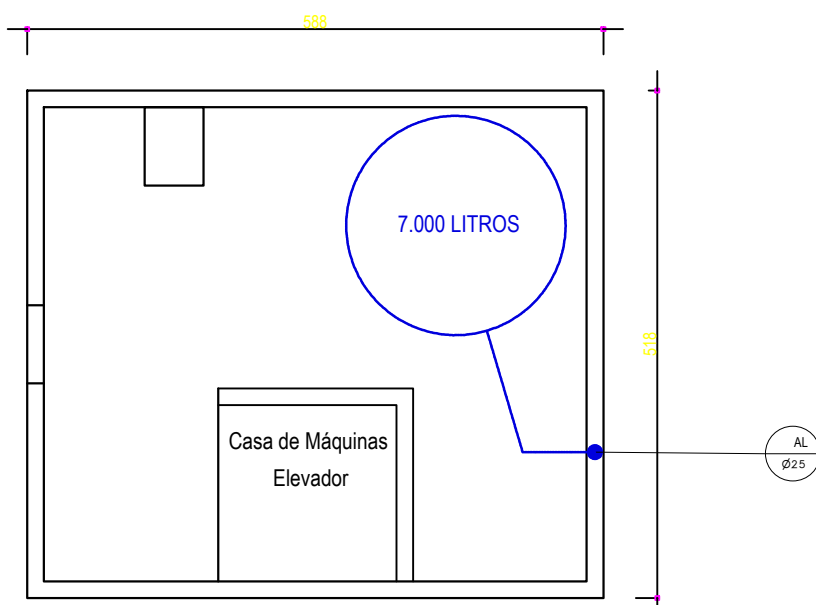
Casa de Máquinas Esc. 1/75
